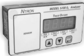
5100氧化锆分析仪 测量范围：0-100% 无消耗氧化锆传感器 应用：制氧机，制氮机
